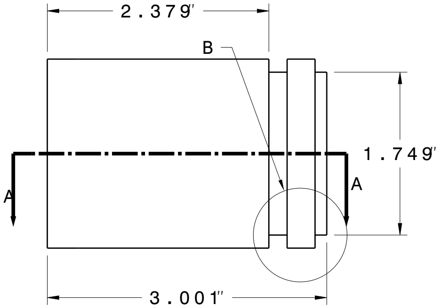
Front view Scale: 1:1
